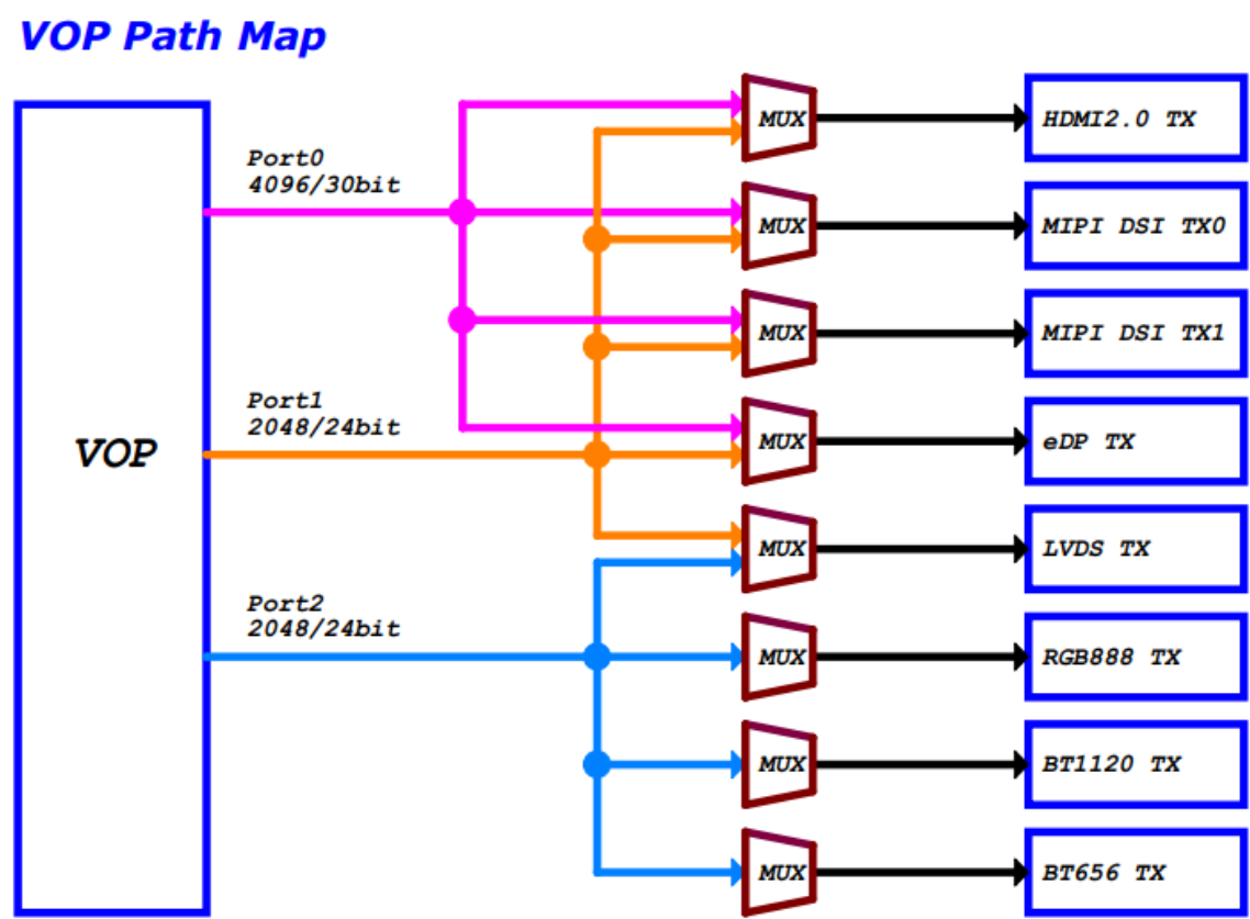
图1 RK3568 VO 输出接口与VoDev连接关系
