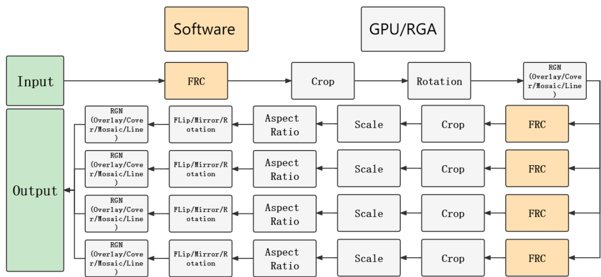
1.3.1 RK356X/RK3588 VPSS USER模式数据流图
